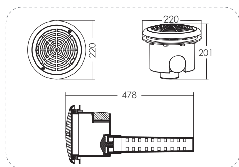
EM2833C/EM2833V
