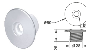
φ2" Face (Standard) Jet
