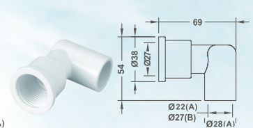
L-Type Jet Body
